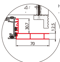
Phần cắt ngang
