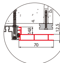
Phần cắt ngang
